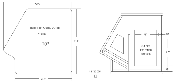
SP400 CPU Ortho Cart
